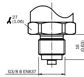
G 3/8 B EN 837
