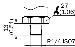
R 1/4 ISO 7
