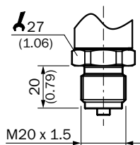
M20 x 1.5
