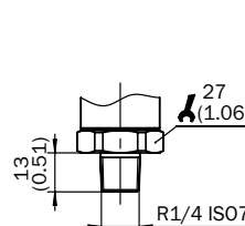
R 1/4 ISO 7
