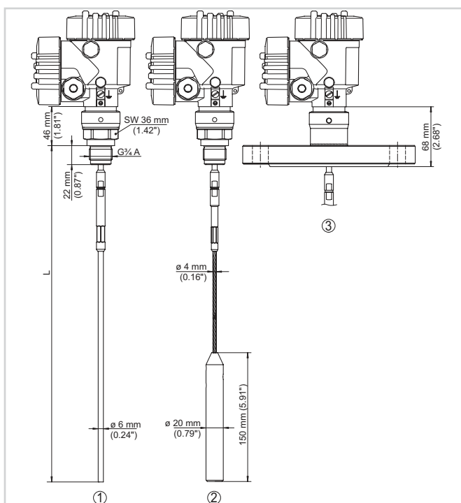
VEGAFLEX 81
