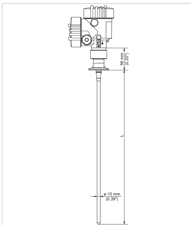
VEGAFLEX 83
