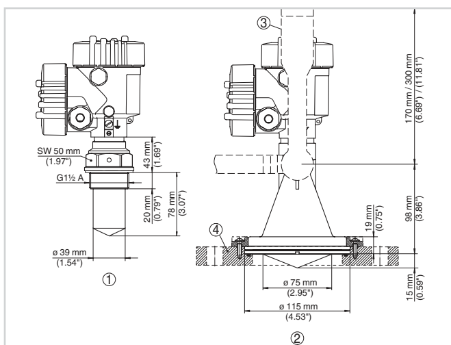
Dimensions VEGAPULS 61
