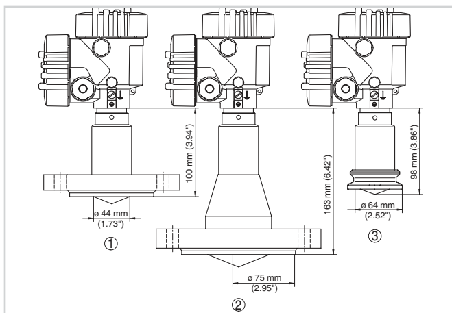
Dimensions VEGAPULS 63
