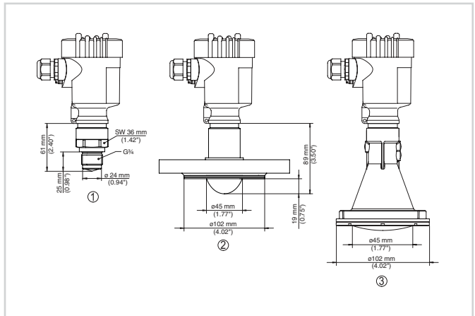
Dimensions VEGAPULS 64
