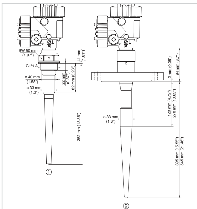
Dimensions VEGAPULS 65
