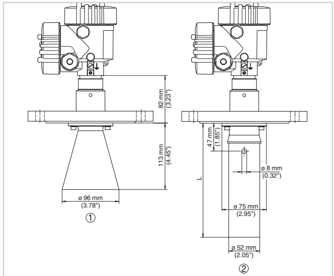
Dimensions VEGAPULS 66
