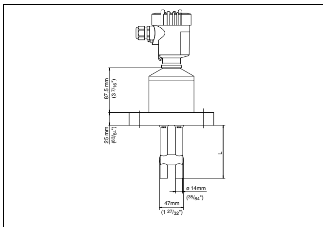
Fig. 21: VEGACAP 69
