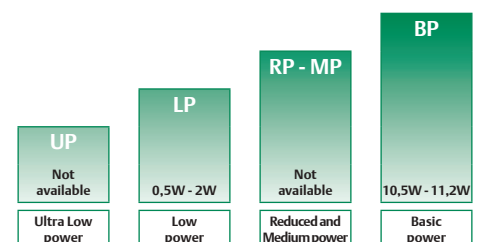
5/3 function
