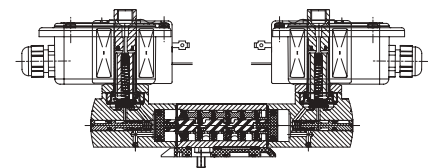
5/3 function
