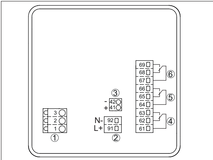
Fig. 9: Wiring plan VEGAMET 341
