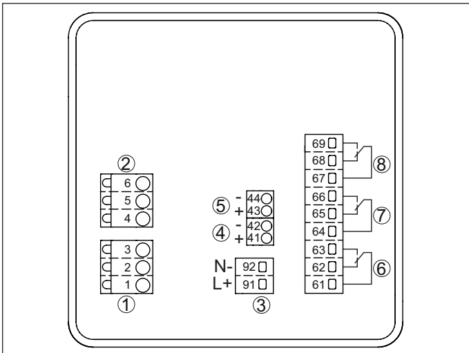
Fig. 10: Wiring plan VEGAMET 342
