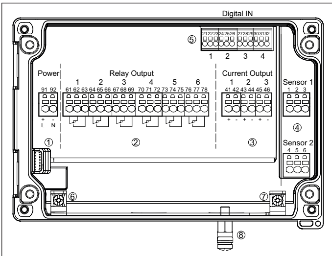
Fig. 14: Wiring plan VEGAMET
